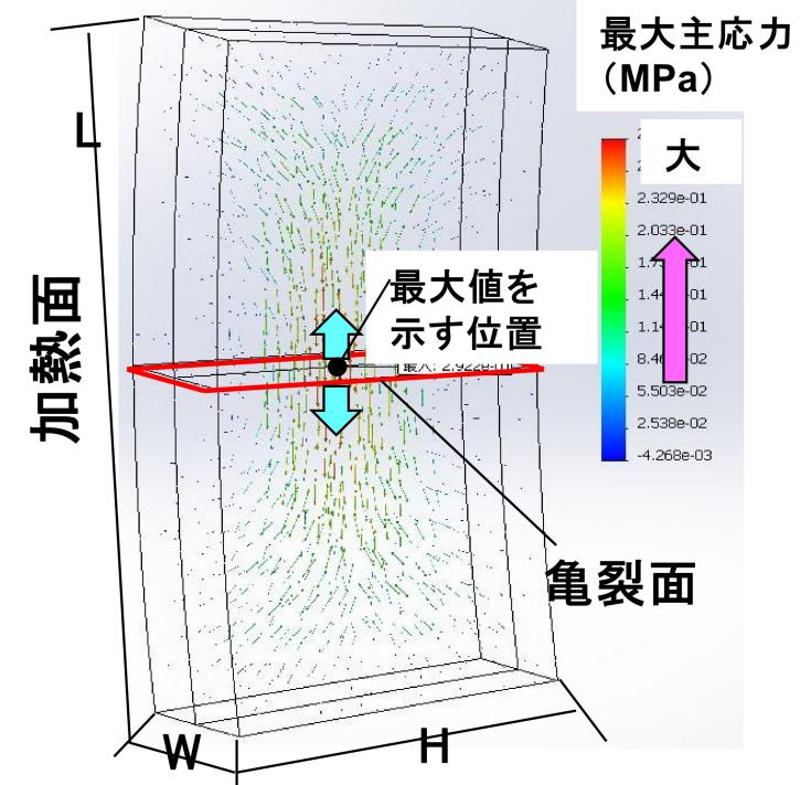
図 2 片面加熱時に生じた最大主応力(引張応力)の分布(図中に小さい矢印群で表示) (図は強調した変形図、 は最も大きな最大主応力を示し、この部位から亀裂が発生する)
