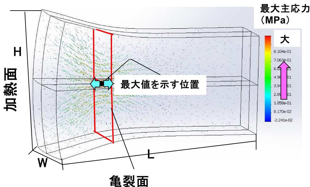
図 2 片面加熱時に生じた最大主応力(引張応力)の分布(図中に小さい矢印群で表示) (図は強調した変形図、 は最も大きな最大主応力を示し、この部位から亀裂が発生する)
